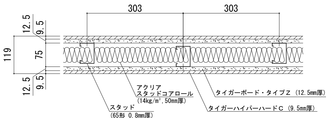
水平断面図（「ハイパーウォールZ・WI アクリア仕様」遮音測定時（S-305-26参照）の壁構造）
